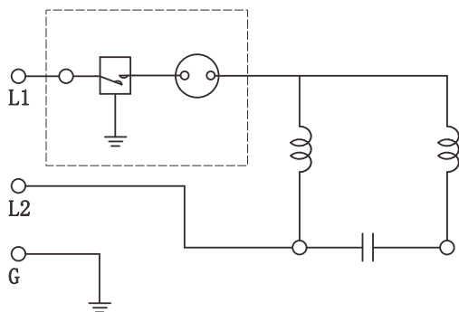
Одна фаза (1)
