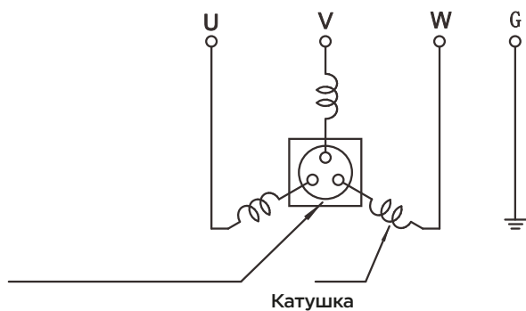
Трехфазный (3)
