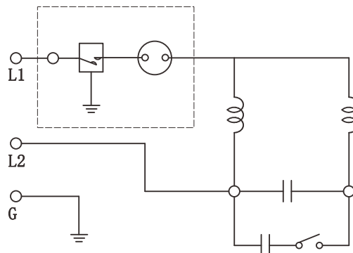
Одна фаза (2)
